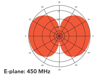
E-plane: 450 MHz
