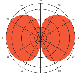
E-plane: 400 MHz
